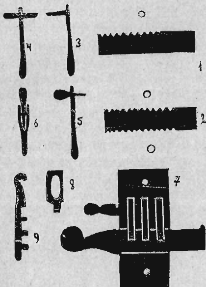
Schemat zamków drewnianych do drzwi.
