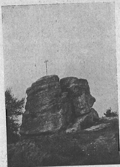
Ciężkowice — Skalka w kształcie baszty.
