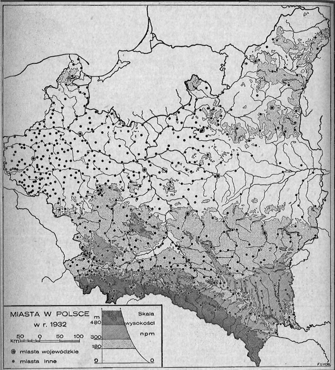
yc. 158. Rozmieszczenie miast w Polsce na tle głównych rysów ukształtowania pionowego powierzchni. Podziałka 1:6,000,000. (Poziomice według „Mapy fizycznej Polski” 1:2 milj. — M. Janiszewskiego).
