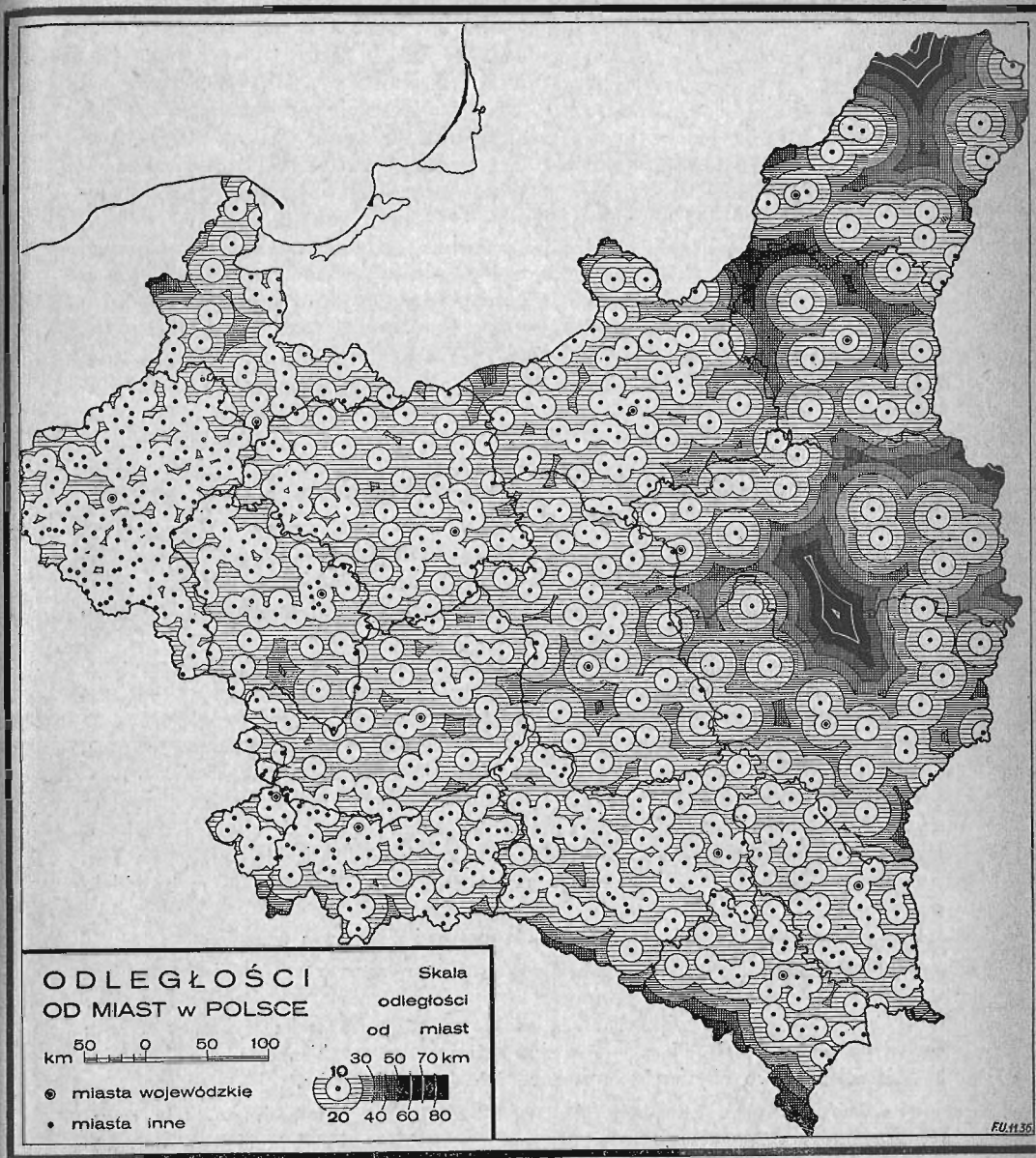
Ryc. 159. Odległości od miast w Polsce strefami 10 kilometrowymi.
